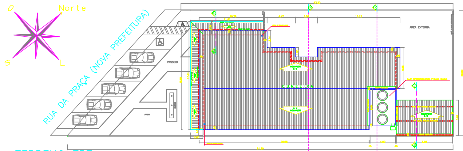
COBERTURA/SITUAÇÃO ESCALA .....1/125
