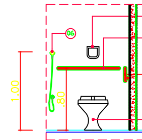
DETALHE 03 (BANCADA EM GRANITO)
